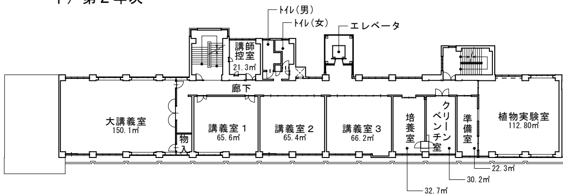
< 2階平面図（第2年次～） >
